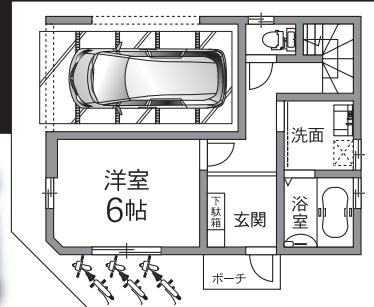
〈Q号地参考プラン〉建物面積/116.49㎡
